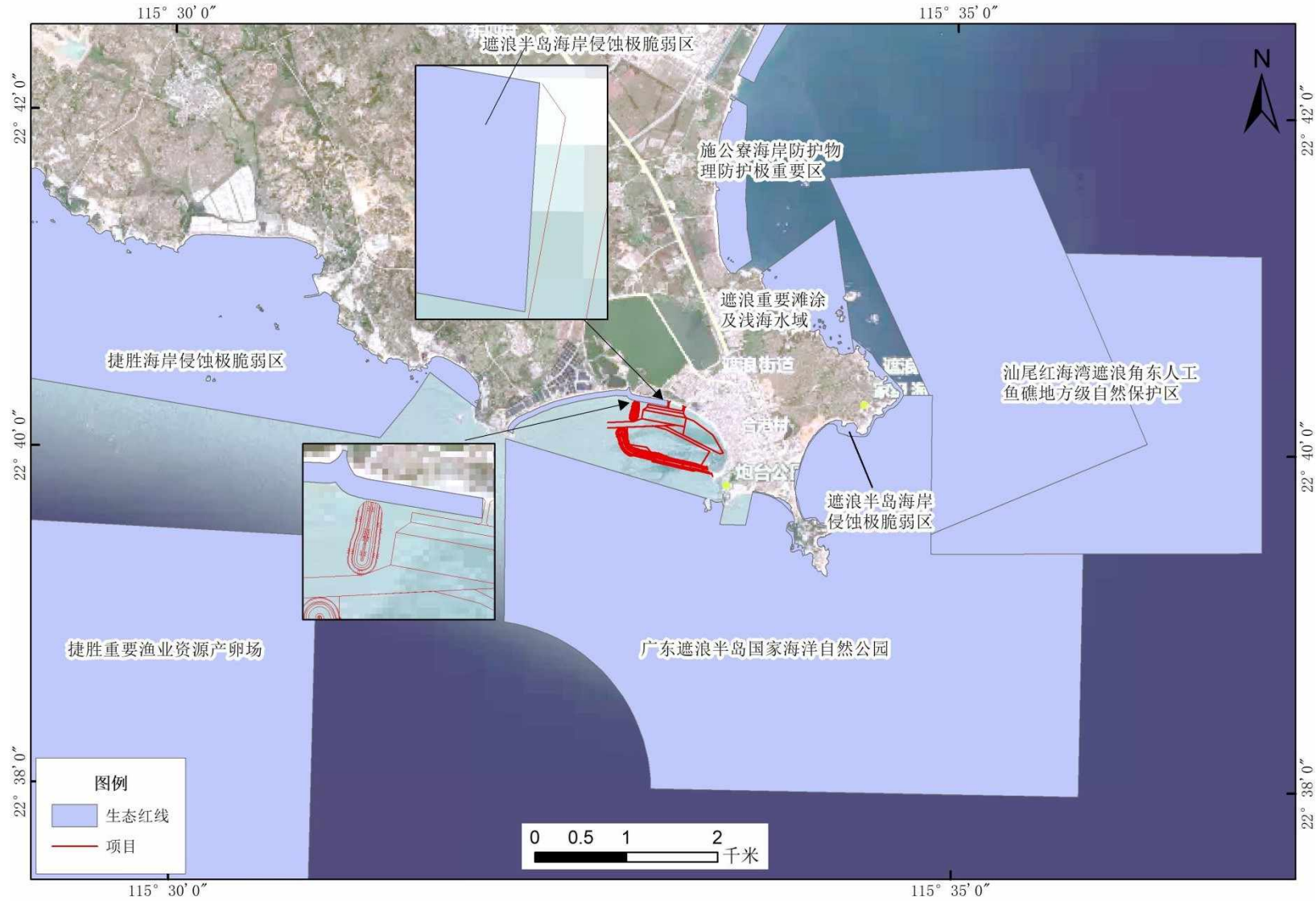
图 11.3.2-1 项目与海洋生态保护红线区位置关系图
