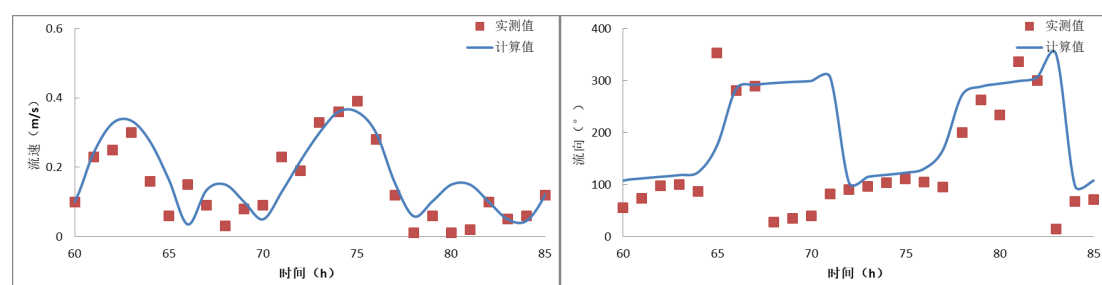
图 8.1.1-7 C2 站流速流向验证图
