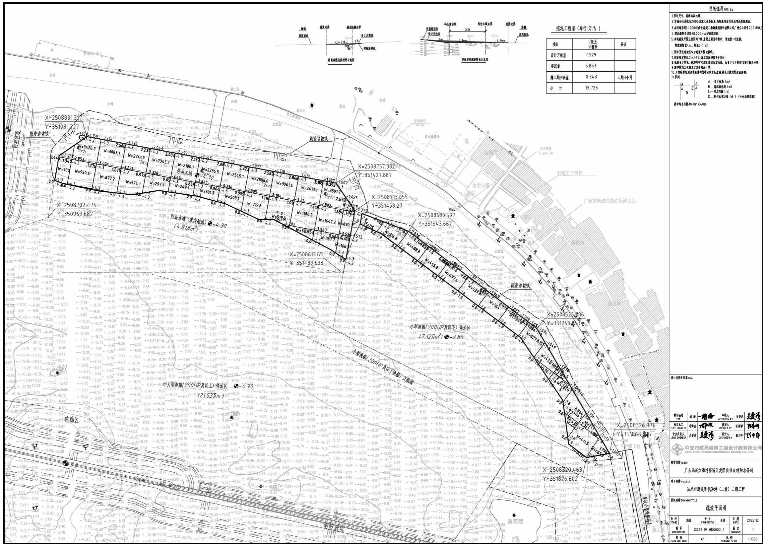
图 4.3-2 项目疏浚范围图
