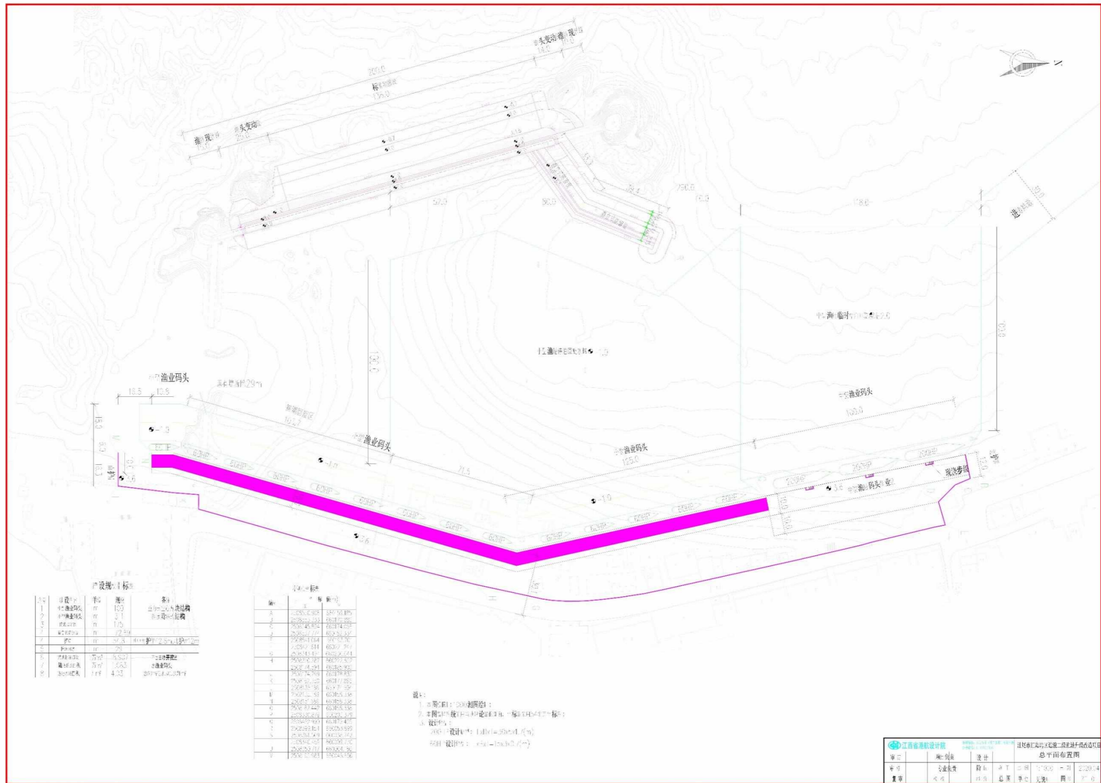
图 3.2-1 一期工程调整后总平面布置图
