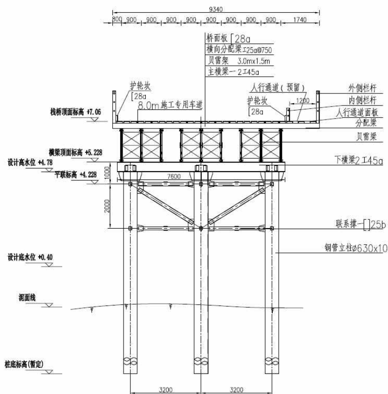
图 4.3.2-14 钢栈桥横剖面图
