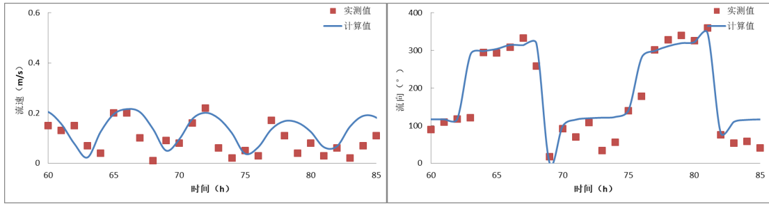
图 8.1.1-10 C5 站流速流向验证图
