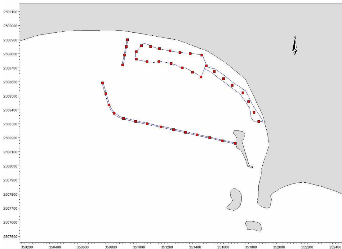
图 8.3.3-1 防波堤、拦砂堤及疏浚区源强点分布图
