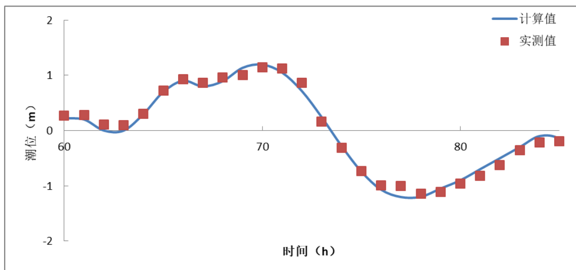
图 8.1.1-5 T2 站潮位验证图
