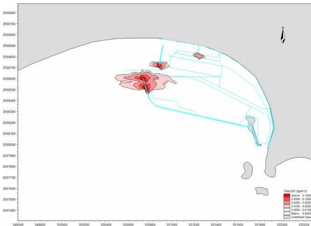
图 8.3.3-8 典型工况 1 悬沙扩散包络线图
