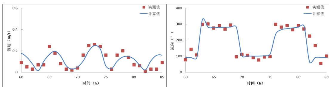
图 8.1.1-8 C3 站流速流向验证图
