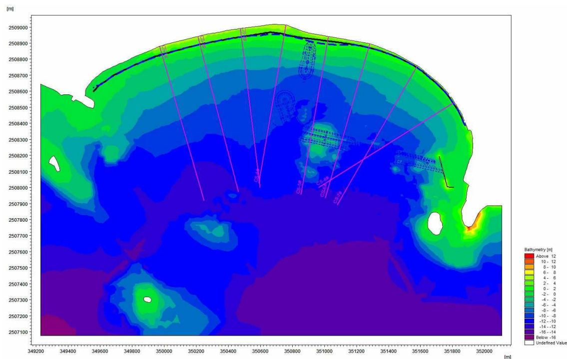
图 8.2.1.4-1 天然条件下 1 年后岸线变化情况
