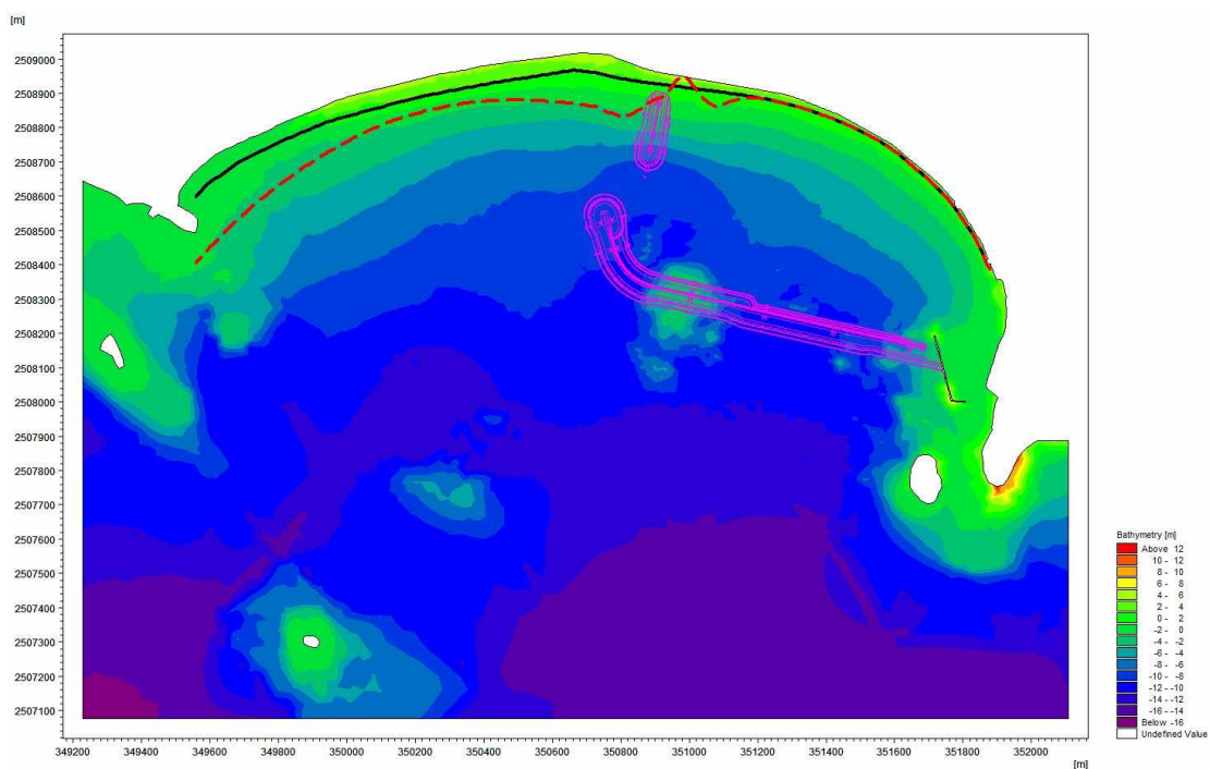
图 8.2.1.5-4 工程实施后 10 年后岸线变化情况
