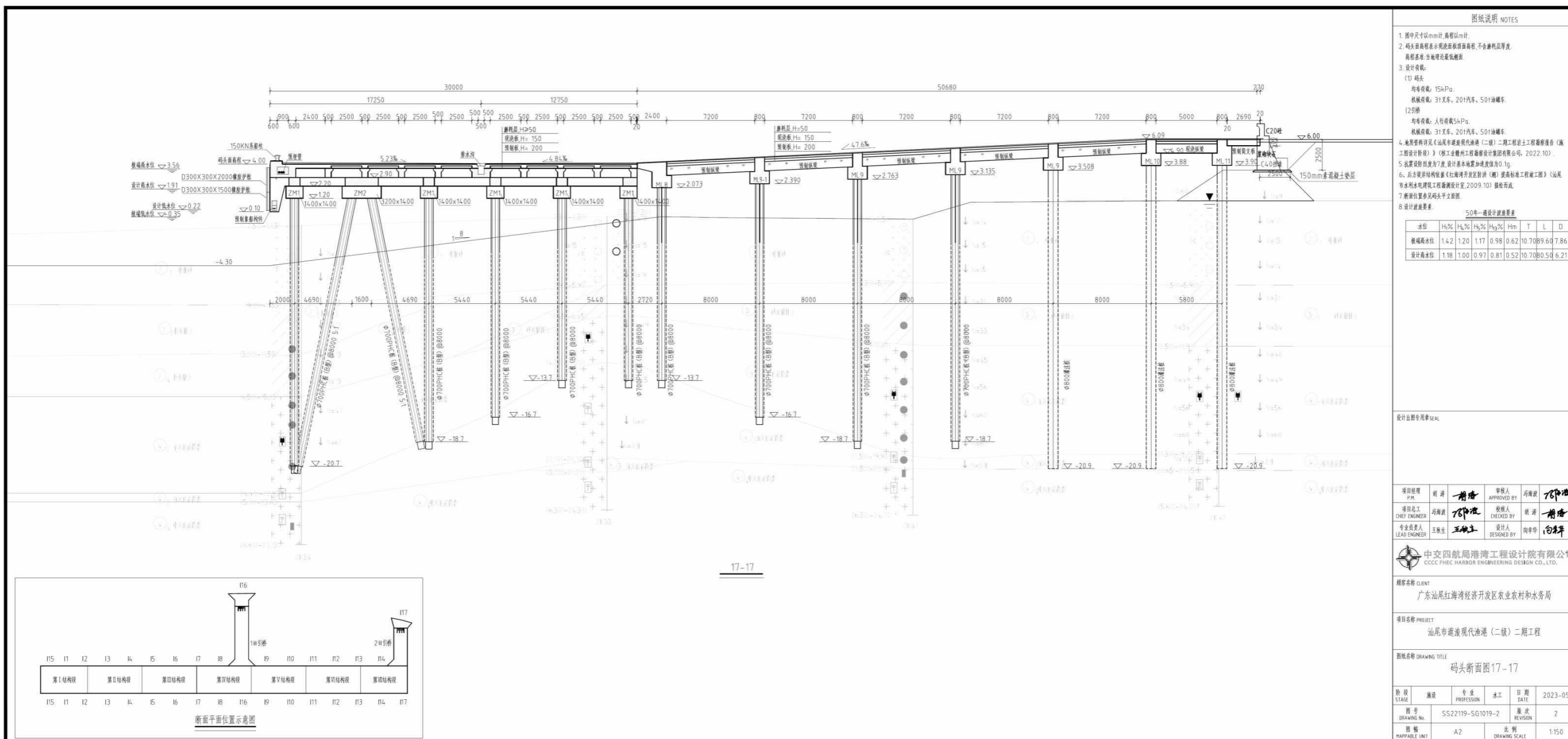
图 4.2.4.1-6 码头结构断面图 17-17
