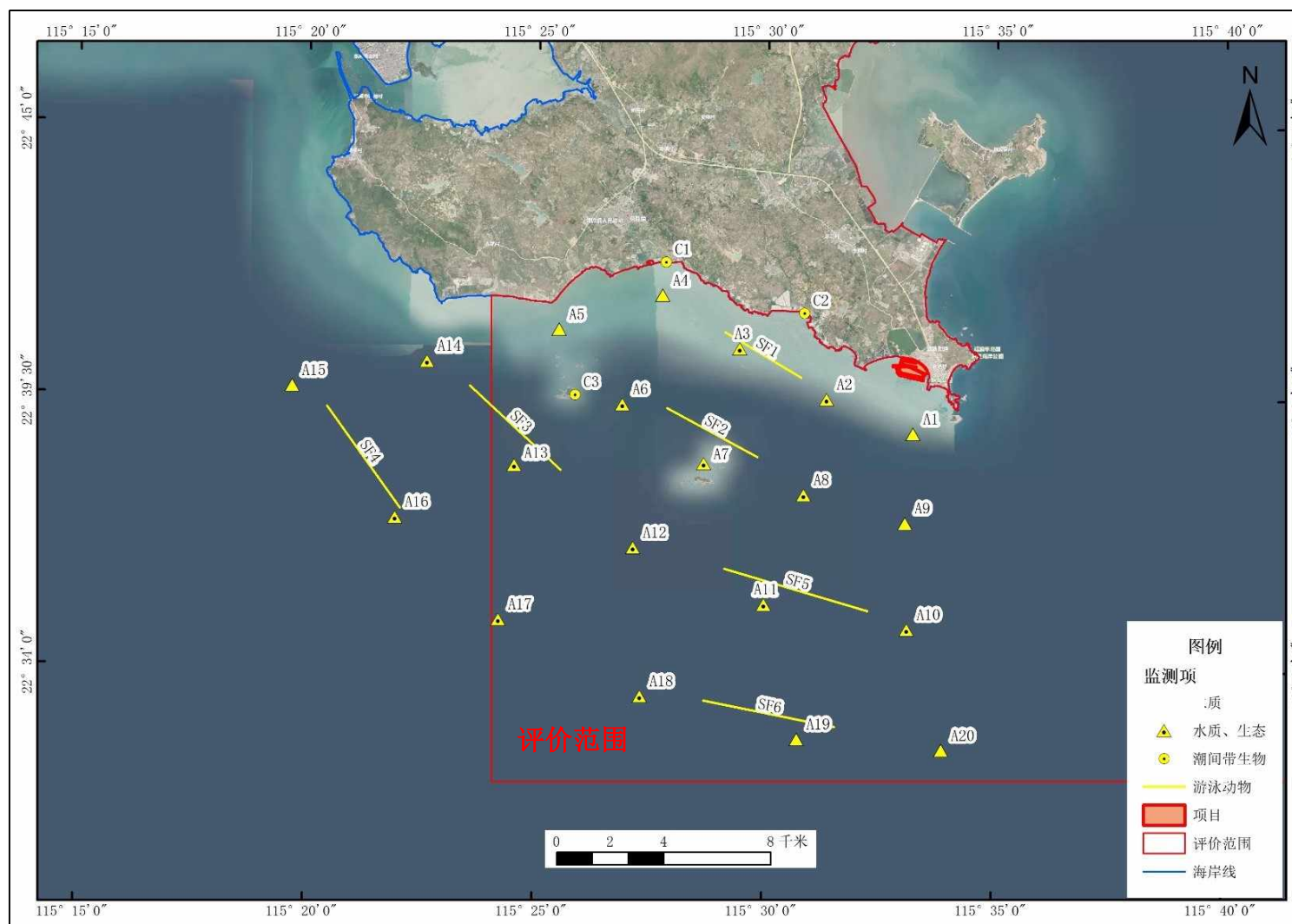
图 7.3.1-2 春季（2021 年 3 月）海洋生态环境调查站位示意图
