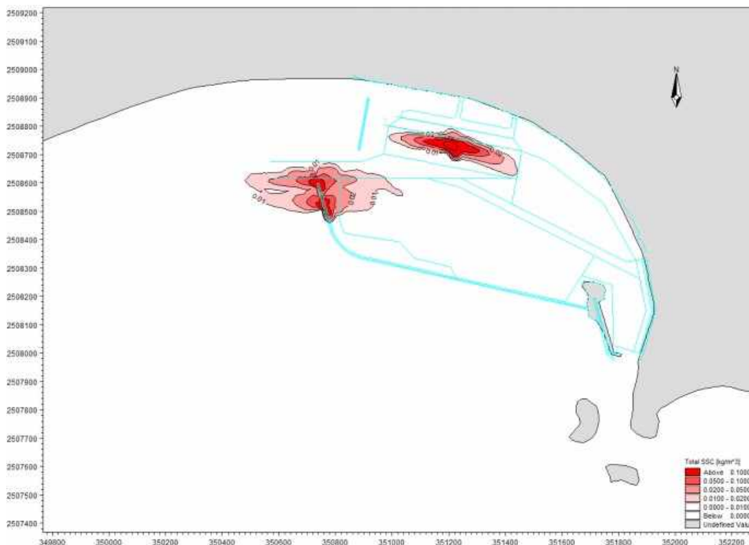
图 8.3.3-9 典型工况 2 悬沙扩散包络线图
