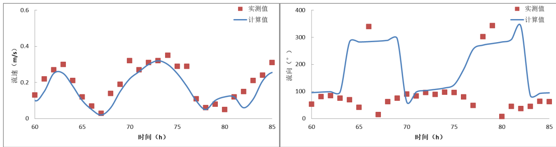
图 8.1.1-11 C6 站流速流向验证图
