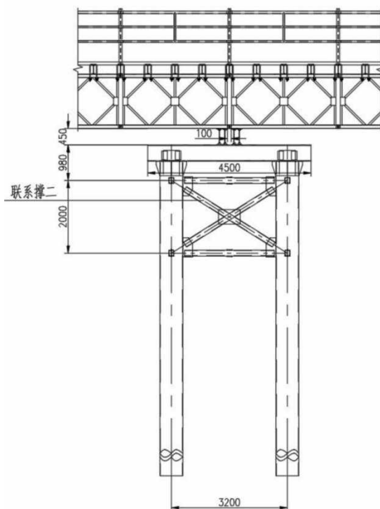
图 4.3.2-15 钢栈桥纵剖面图
