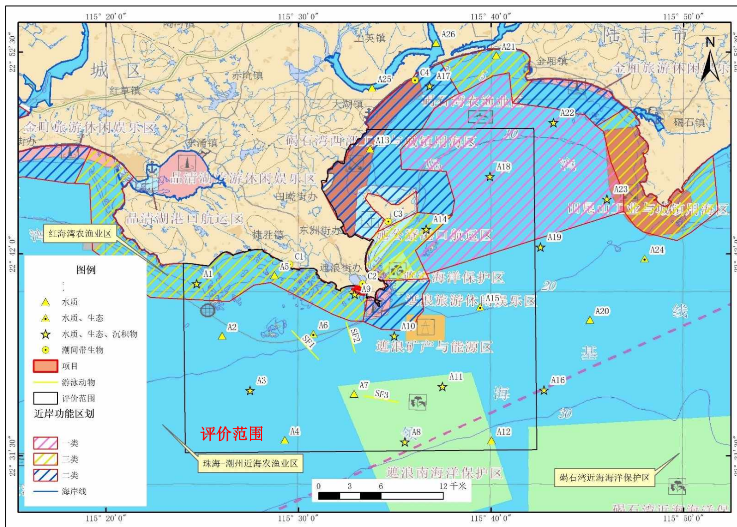
图 7.3.3-3 春季（2022 年 4 月）调查站位所在海洋功能区及近岸海域环境功能区示意图
