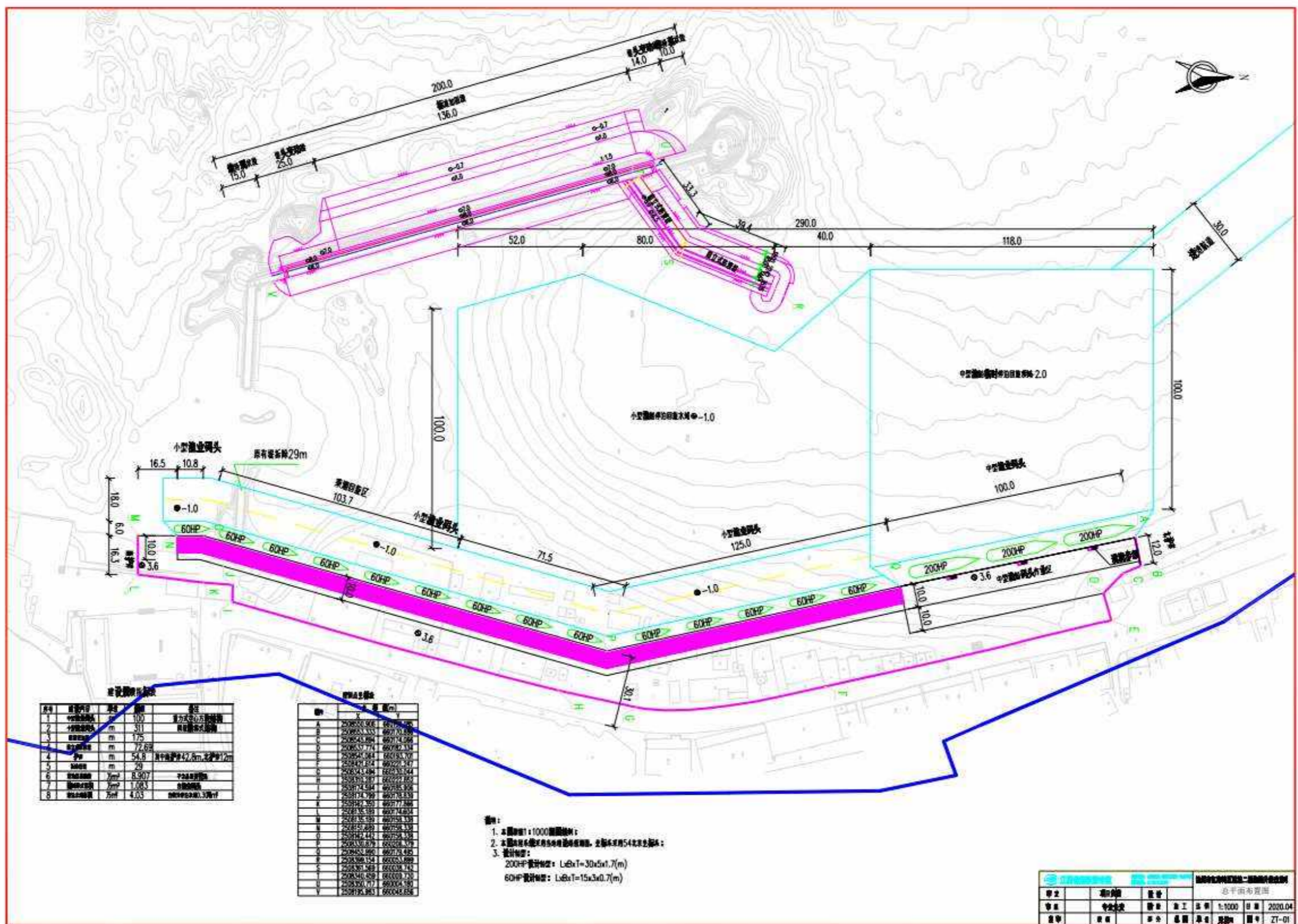
图 3.2-2 一期工程平面布置与 2012 年广东海岸线位置关系图
