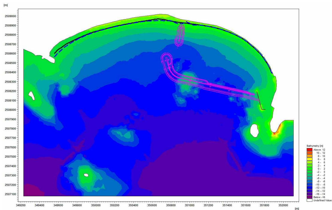
图 8.2.1.5-1 工程实施后 1 年后岸线变化情况
