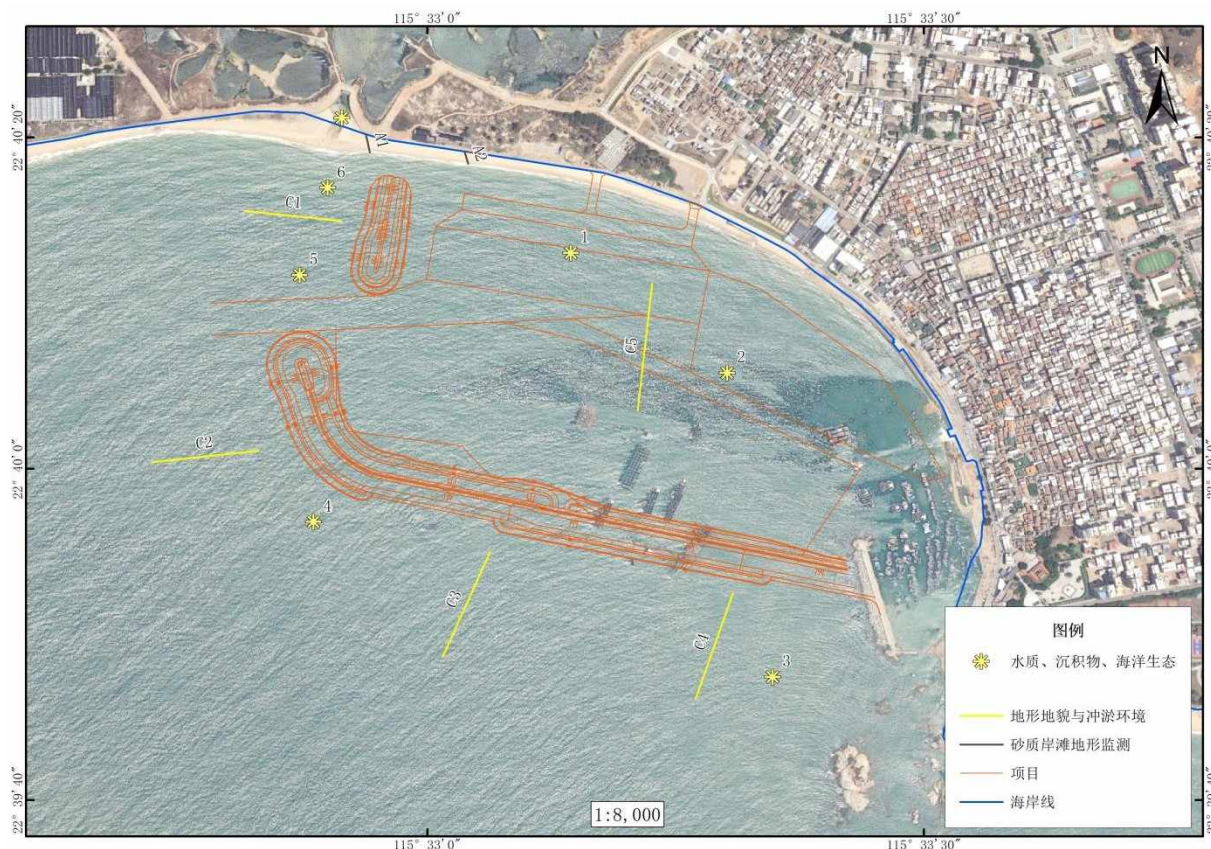
图 13.4.1-2 海洋环境跟踪监测站位图
