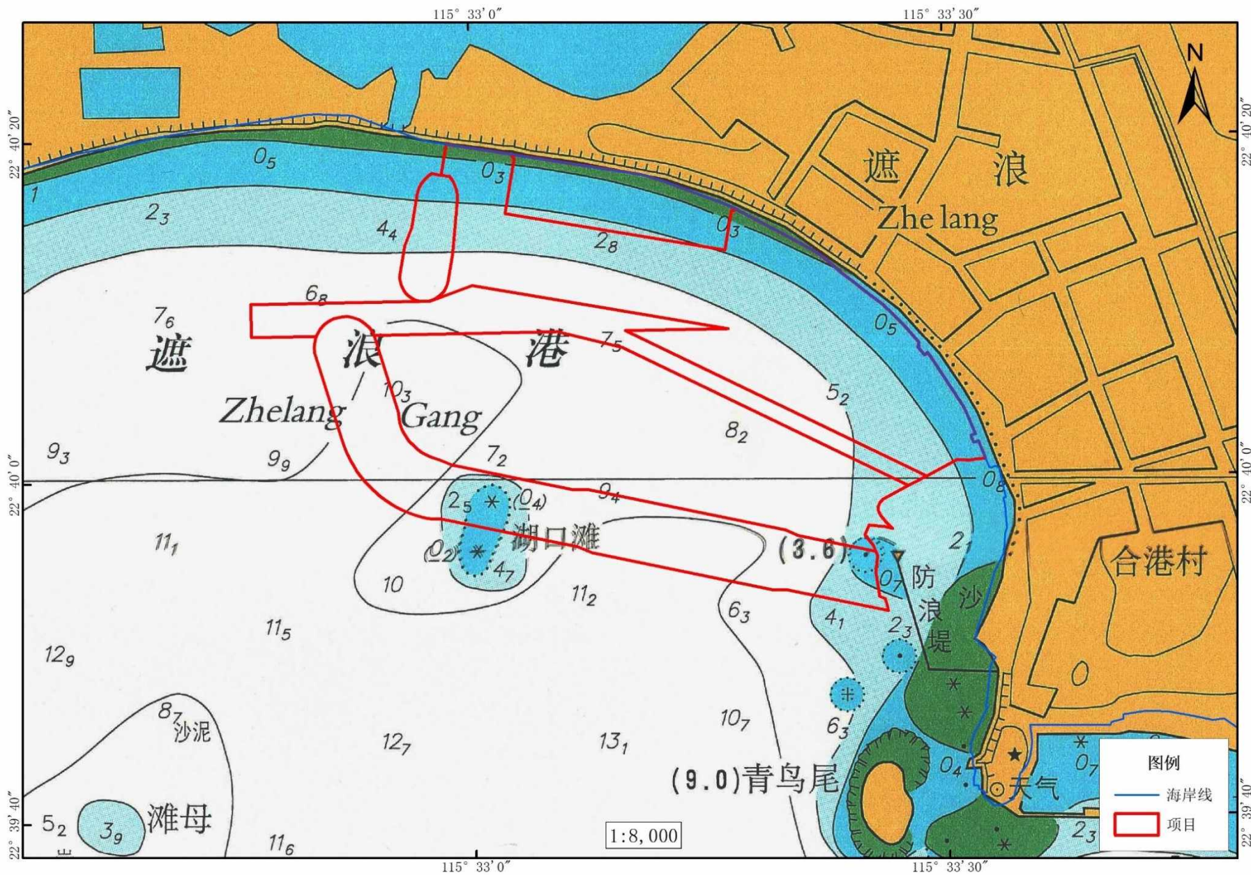
图 7.2.3-1 现状下工程近岸水深形势图
