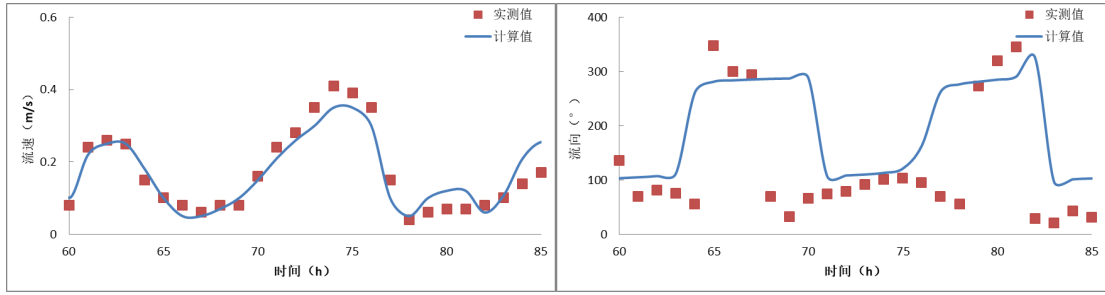
图 8.1.1-9 C4 站流速流向验证图
