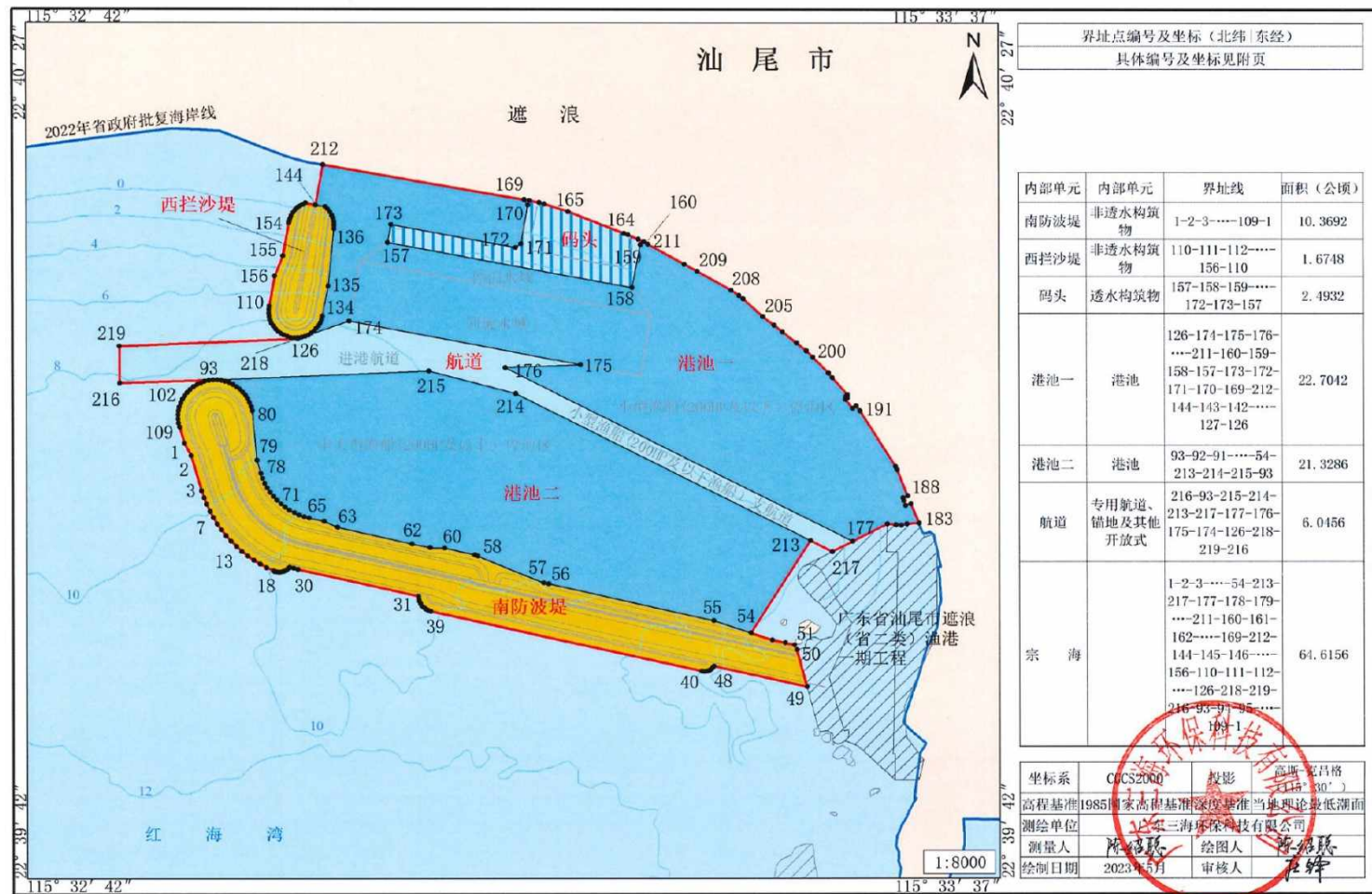
汕尾市遮浪现代渔港（二级）二期工程宗海界址图
