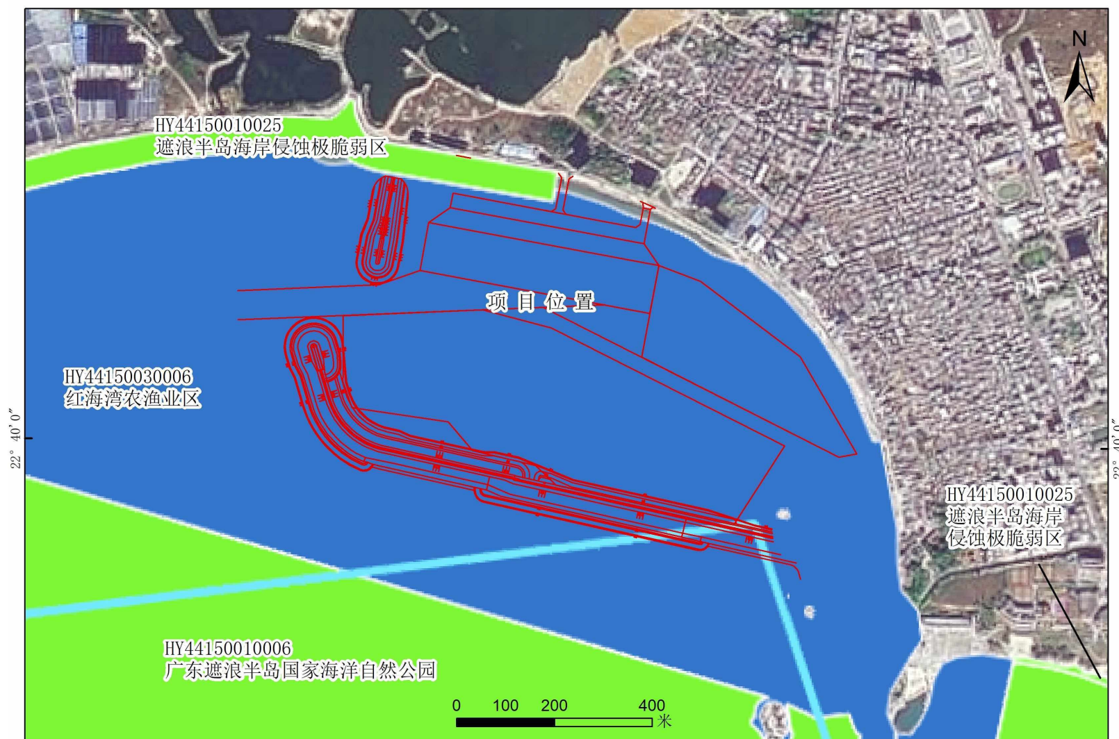
图 2.3.8-1 项目与广东三线一单平台截图叠加示意图
