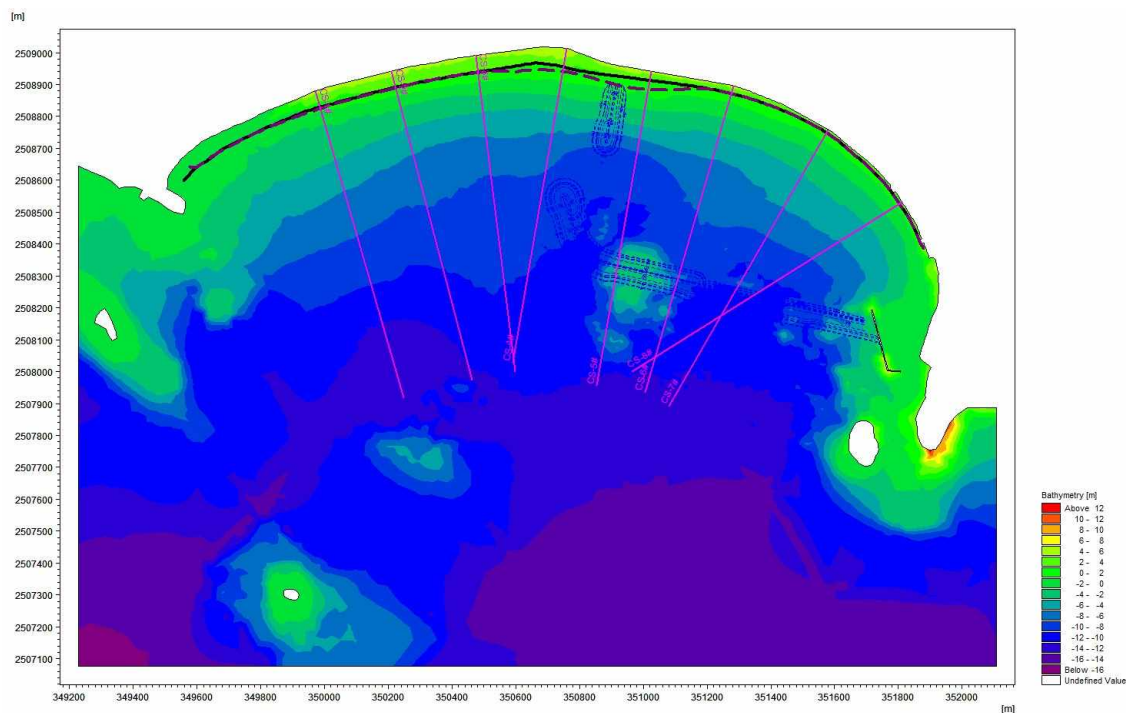
图 8.2.1.4-2 天然条件下 2 年后岸线变化情况
