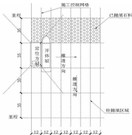
图 4.3.2-9 基床抛石网格定位示意图（单位：m）
