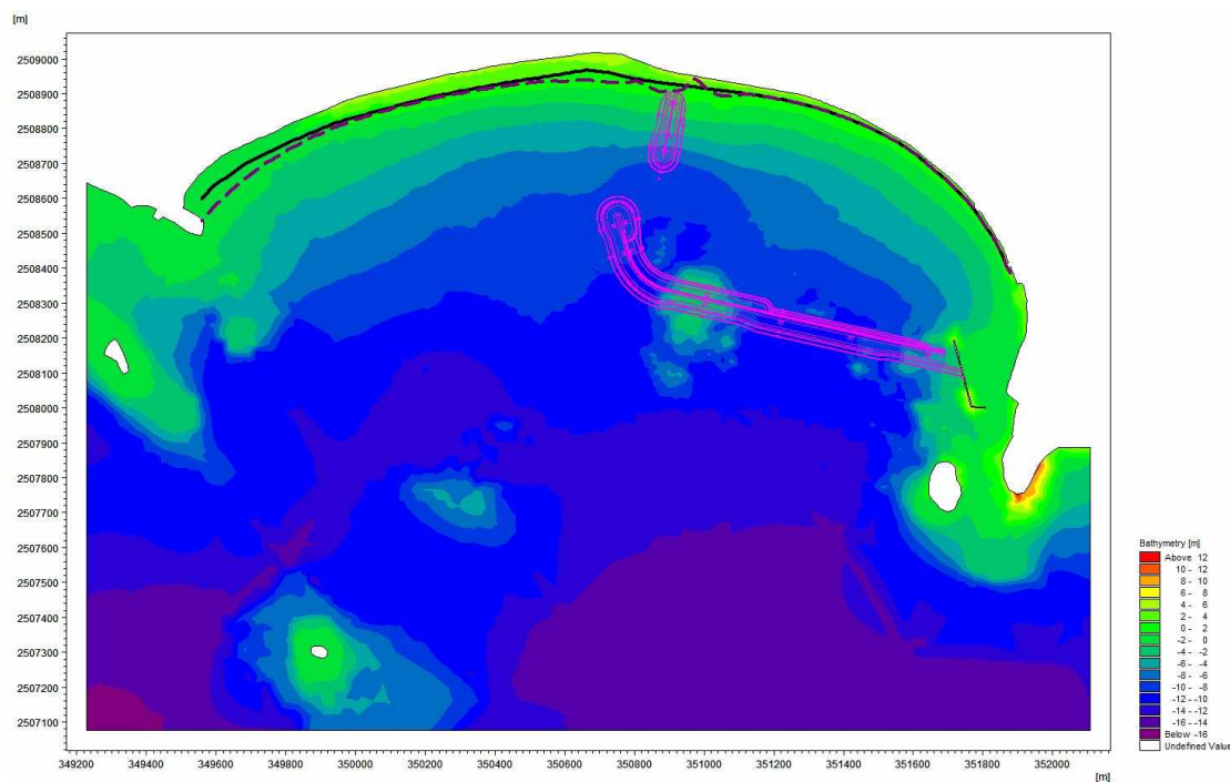
图 8.2.1.5-2 工程实施后 2 年后岸线变化情况
