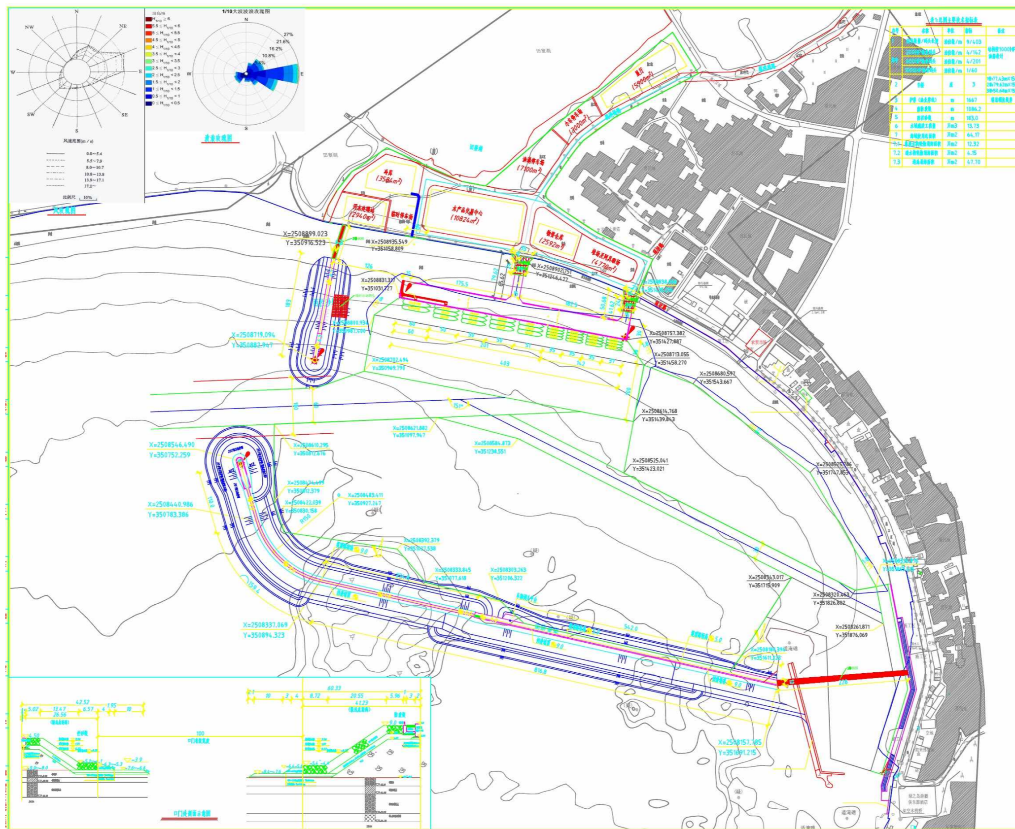
4.3.2-1 施工总平面布置图
