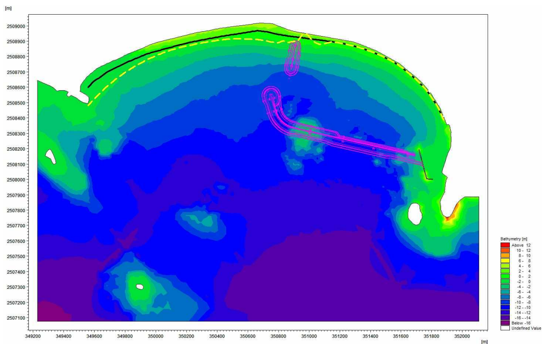
图 8.2.1.5-3 工程实施后 5 年后岸线变化情况
