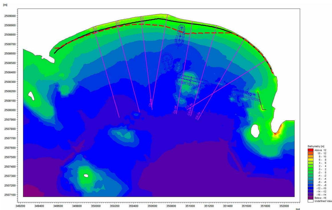
图 8.2.1.4-4 天然条件下 10 年后岸线变化情况
