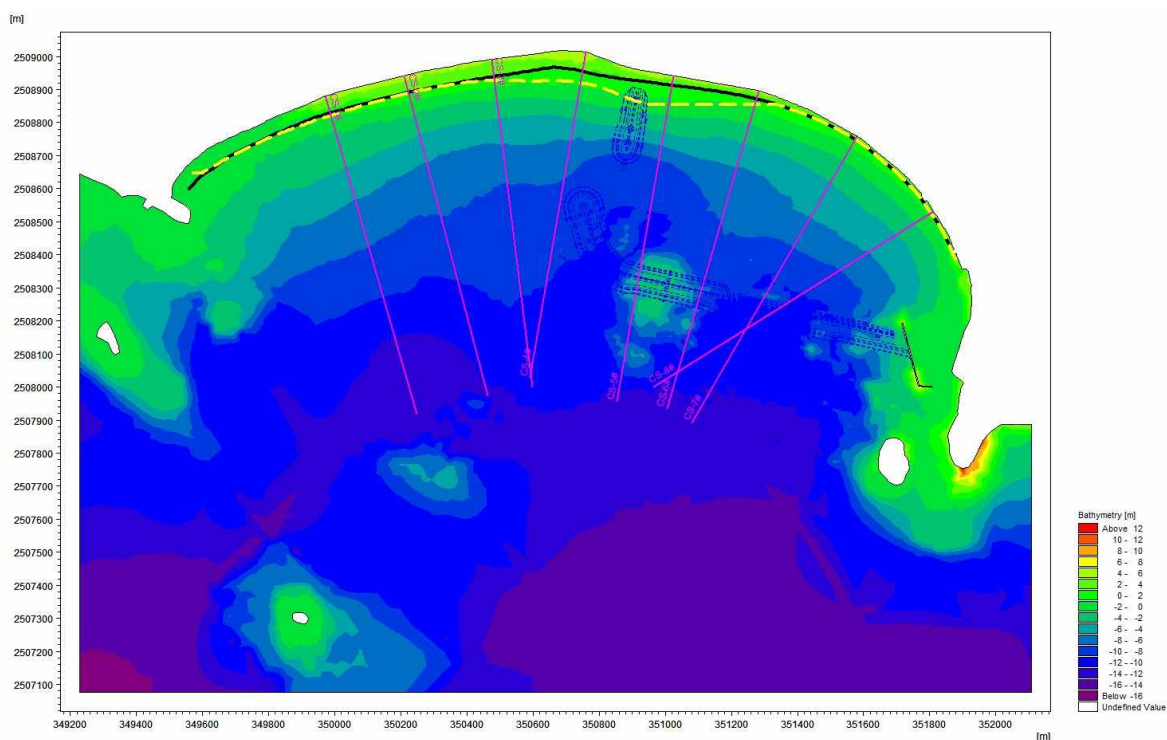
图 8.2.1.4-3 天然条件下 5 年后岸线变化情况
