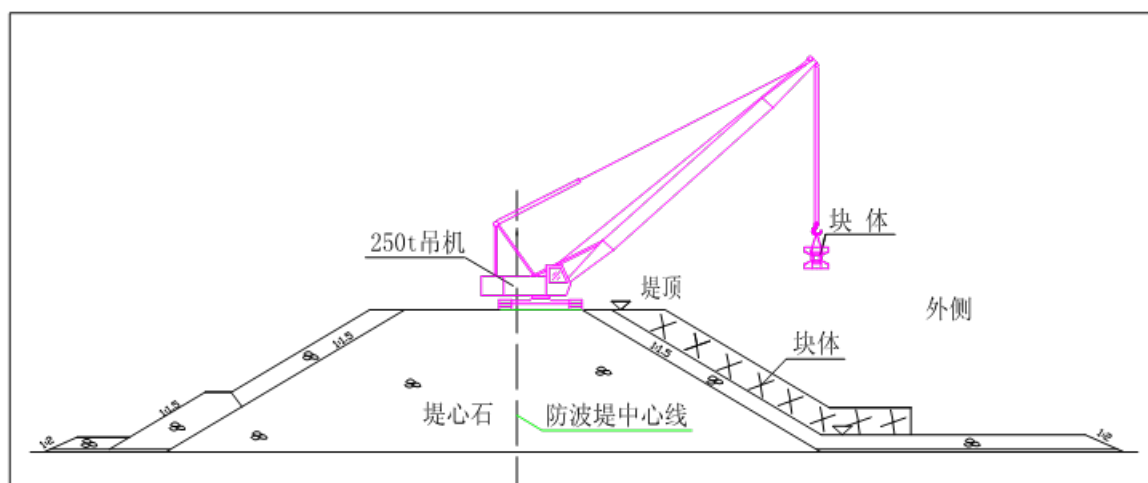
图 4.3.2-12 扭王字块安装示意图
