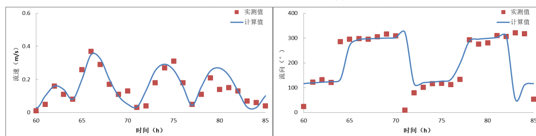
图 8.1.1-6 C1 站流速流向验证图
