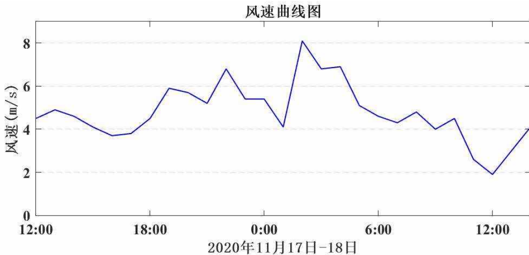
图 7.1.1.2-1 C4 站位风速风向过程曲线
